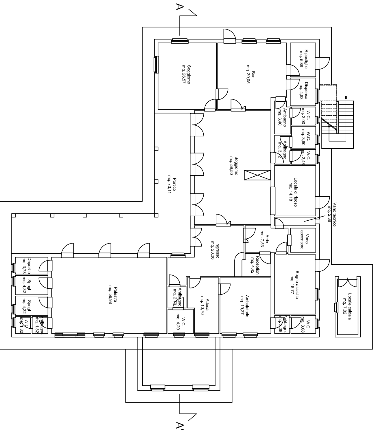
Stato confronto: pianta
